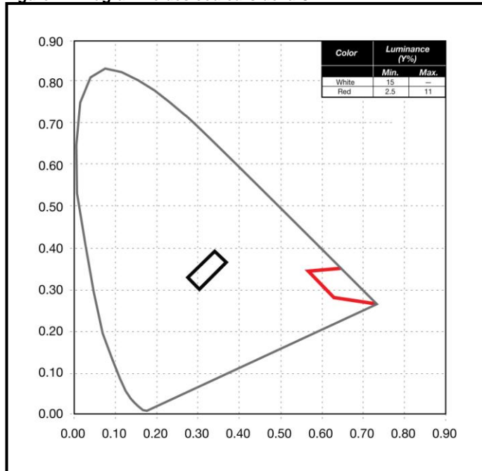
Figure A : Diagramme des couleurs de la CIE
