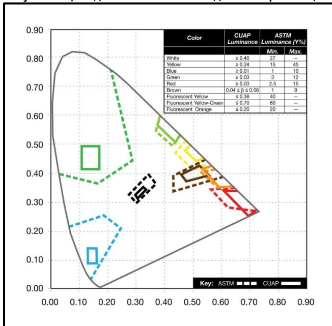
Рисунок А: Цвет для использования в дневное время – цветовая схема CIE
